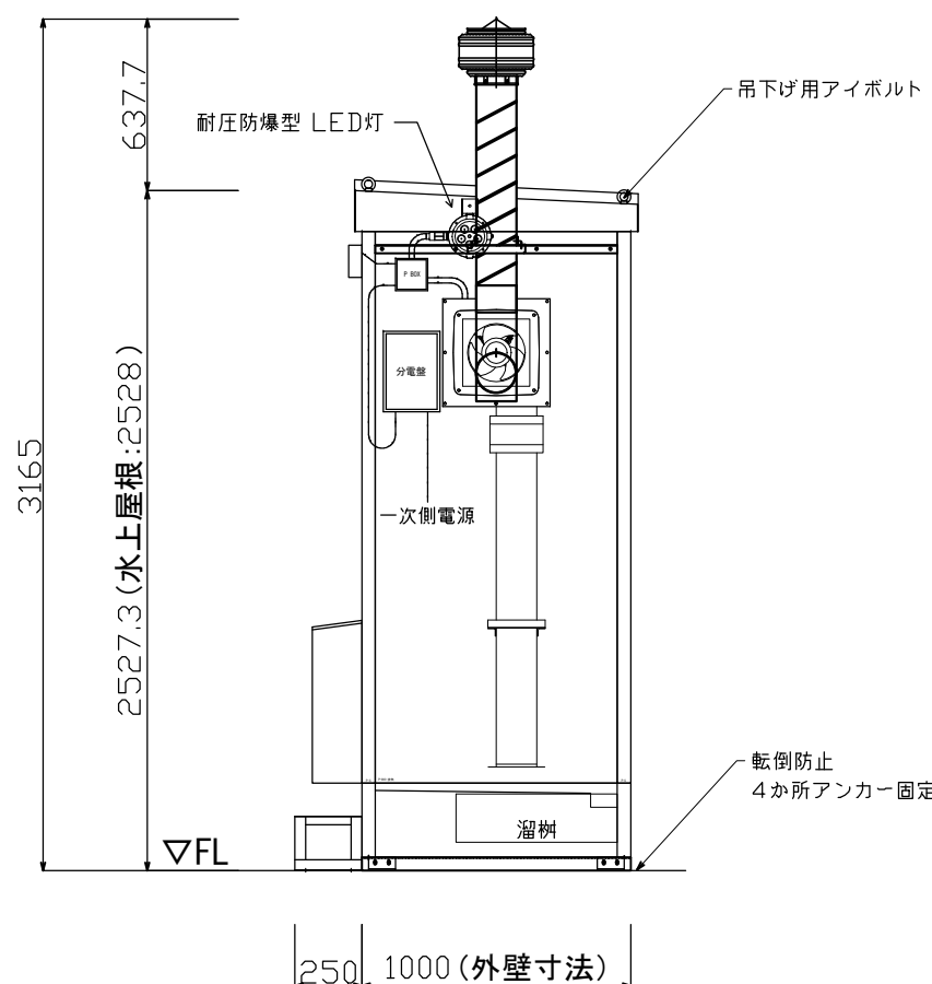
右側面図
